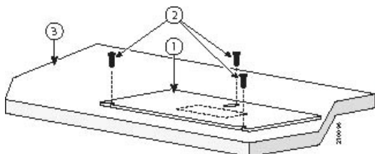
Figure 1 Positionnement du gabarit et insertion des vis
