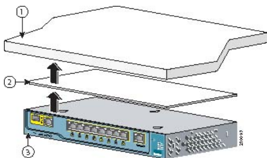
Figure 3 Montage du commutateur avec un panneau aimanté
