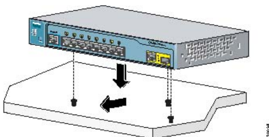
Figure 2 Placement du commutateur sur les vis de montage
