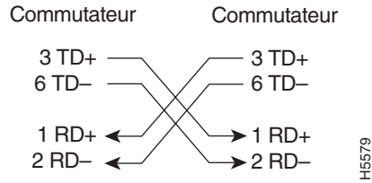
Figure B-6 Schéma de câble croisé à deux paires torsadées pour les ports 10/100
