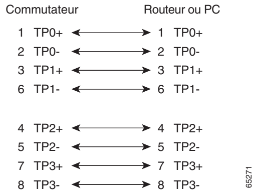
Figure B-7 Schéma de câble direct à quatre paires torsadées pour les ports 1000BASE-T
