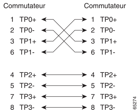
Figure B-8 Schéma de câble croisé à quatre paires torsadées pour les ports 1000BASE-T
