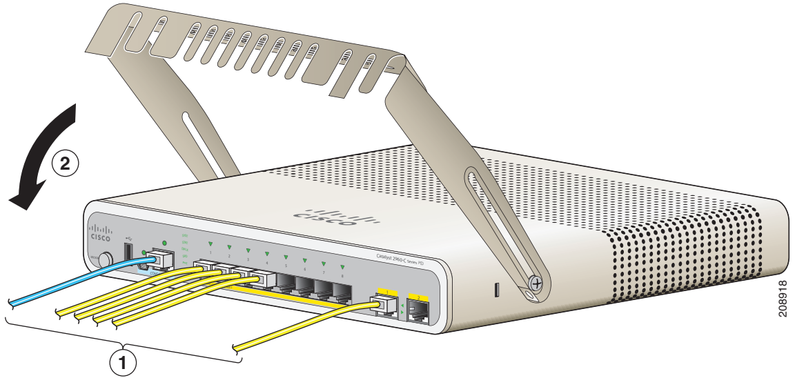
Figure 2-24 Fixation des câbles au commutateur
