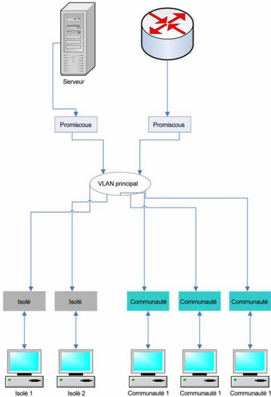
Figure 2 Trafic des serveurs/routeurs vers les hôtes
