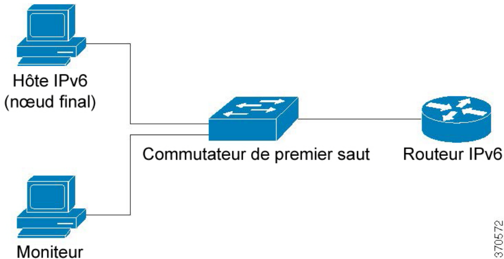
Figure 6 Configuration de la Sécurité du premier saut IPv6
