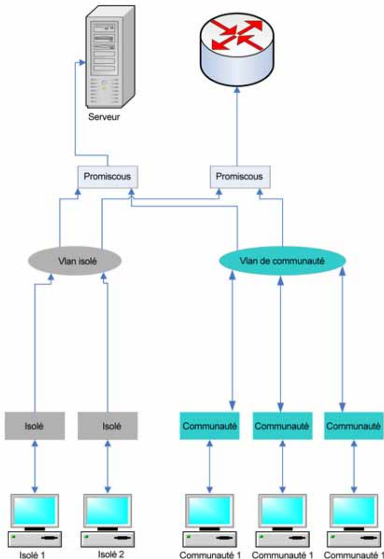
Figure 1 Trafic des hôtes vers les serveurs/routeurs
